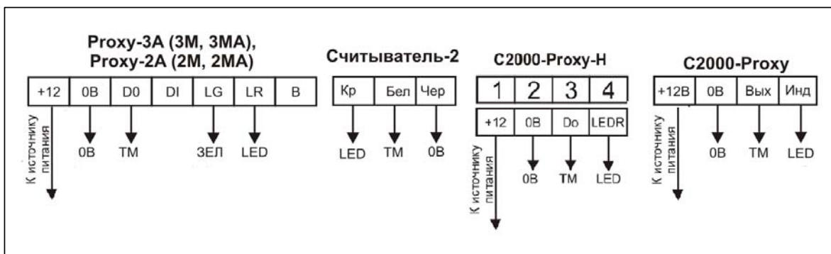
Рисунок 7. Подключение считывателей
