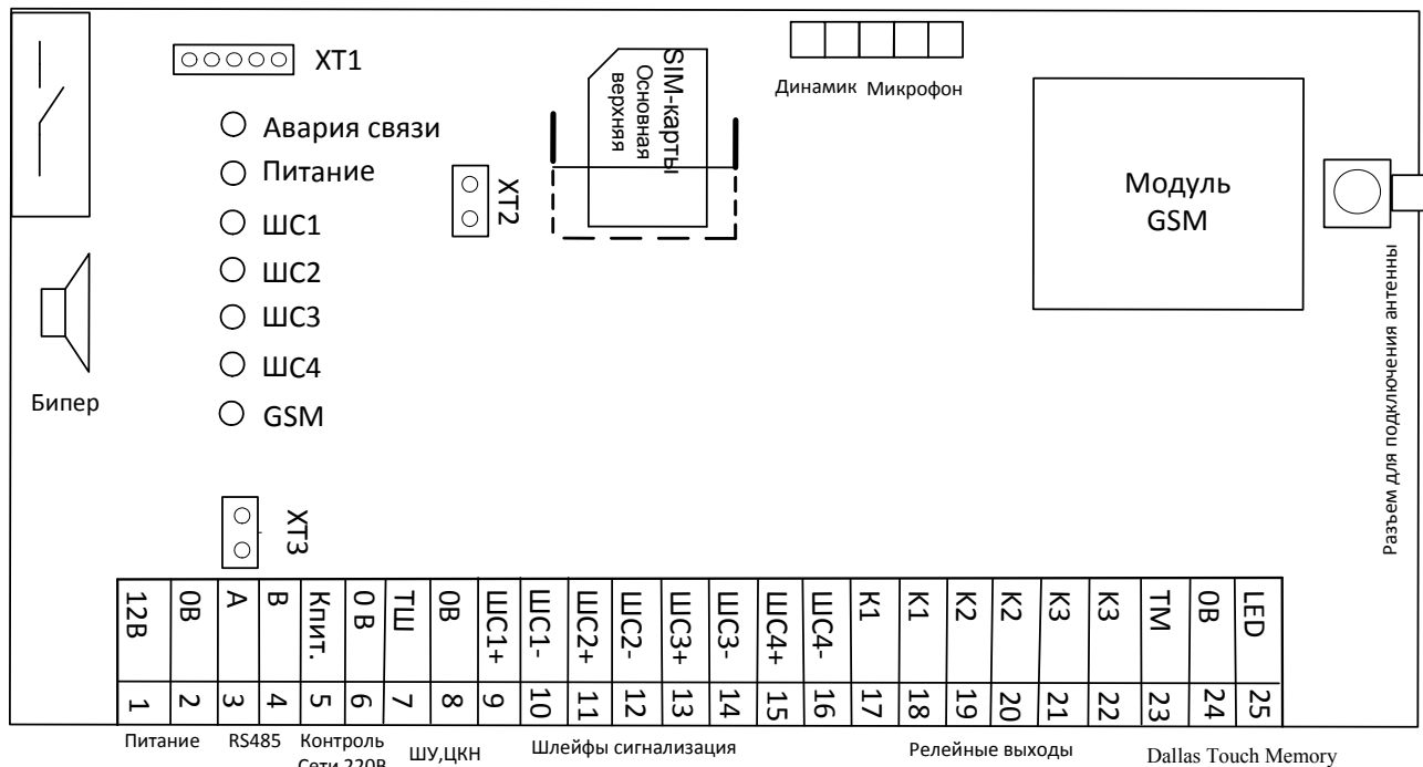
Рисунок 1. Блок схема «УО-4С»
