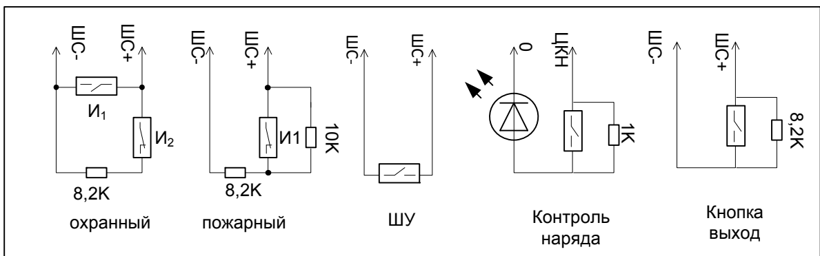
Рисунок 6. Подключение ШС, ШУ
