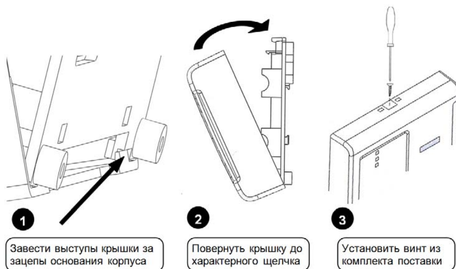
Рисунок 8. Монтаж крышки
