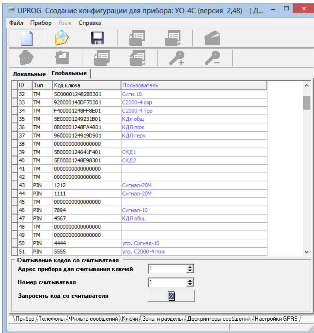
Рисунок 18. Глобальные ключи, мастер режим
