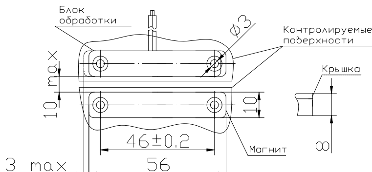
Рисунок 2 Установочные размеры
