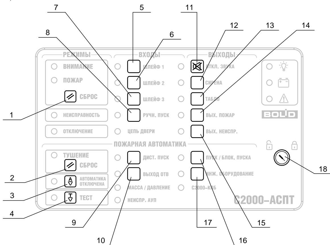
Рисунок 2. Расположение кнопок
