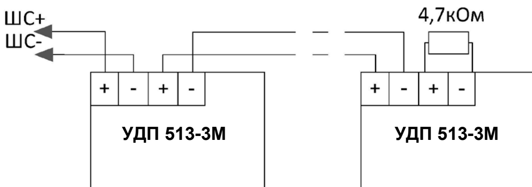
Схема подключения извещателей «УДП 513-3М» ко входу дистанционного пуска
