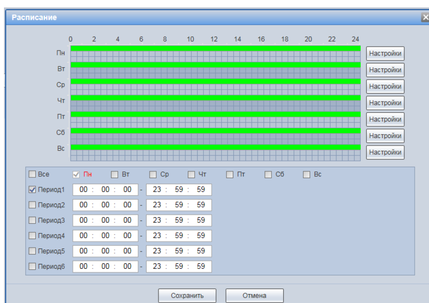
Рисунок 7.79 – Вкладка «Изменение сцены»: Расписание
