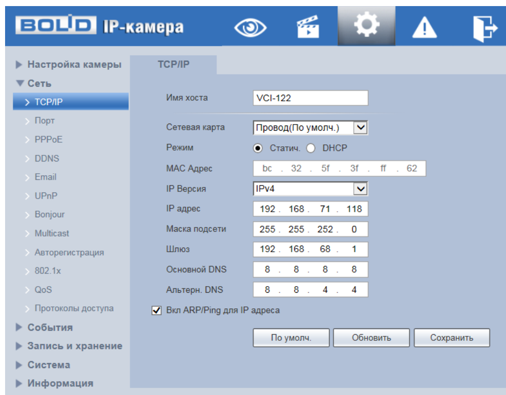
Рисунок 7.52 – Подпункт меню «TCP/IP»
