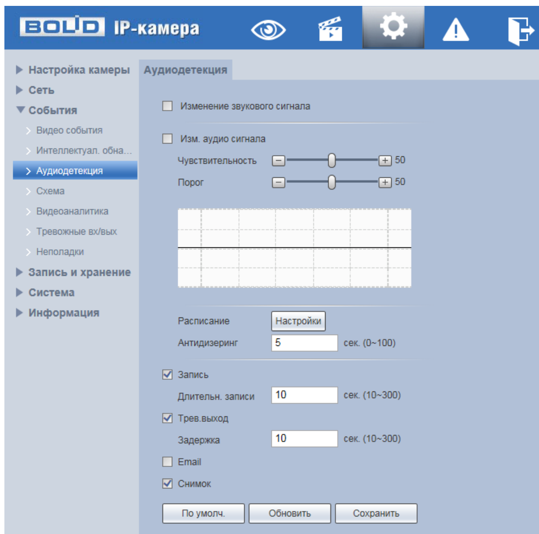
Рисунок 7.81 – Подпункт меню «Аудиодетекция»
