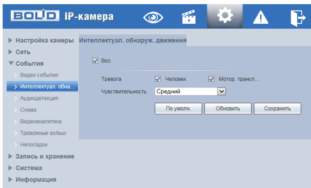
Рисунок 7.80 – Подпункт меню «Интеллектуальное обнаружение движения»
