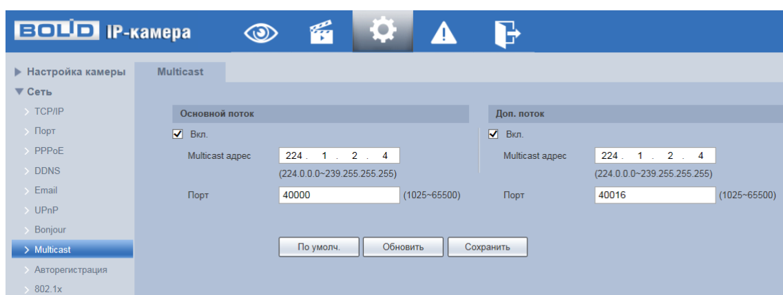
Рисунок 7.63 – Подпункт меню «Multicast»
