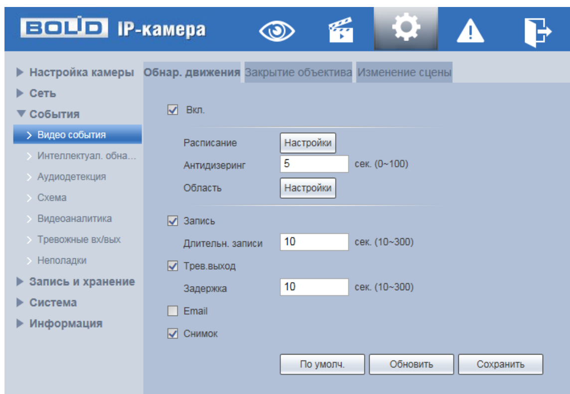
Рисунок 7.73 – Вкладка «Обнаружение движения»
