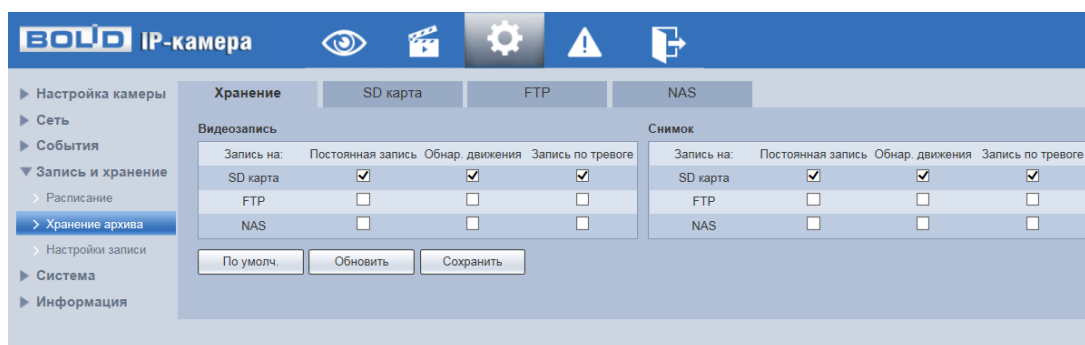
Рисунок 7.101 – Вкладка «Хранение»
