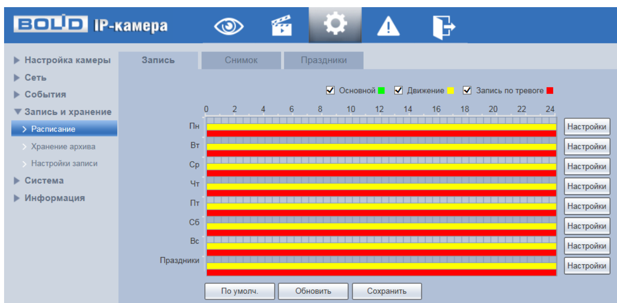
Рисунок 7.95 – Вкладка «Запись»
