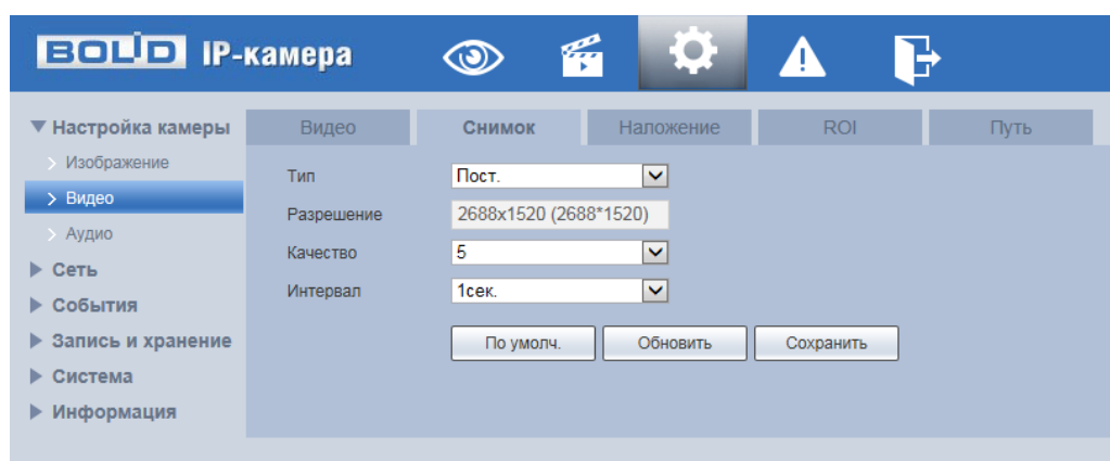
Рисунок 7.39 – Вкладка «Снимок»
