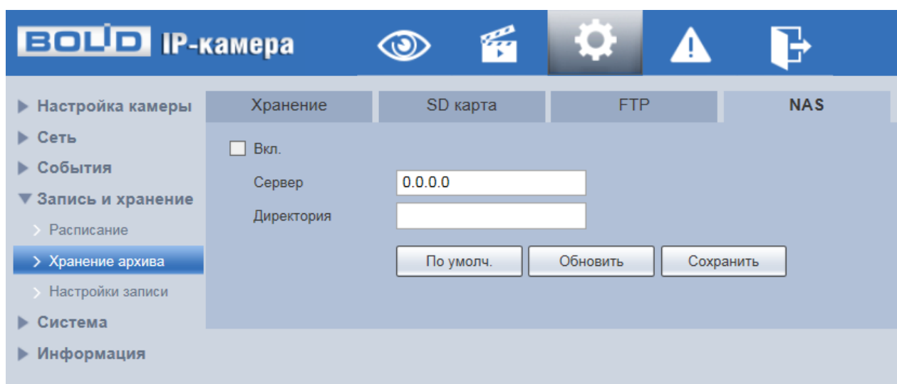
Рисунок 7.104 – Вкладка «NAS»
