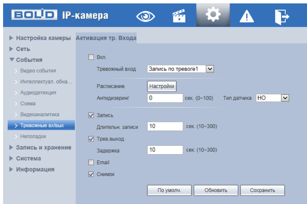
Рисунок 7.86 – Подпункт меню «Тревожные входы/выходы»
