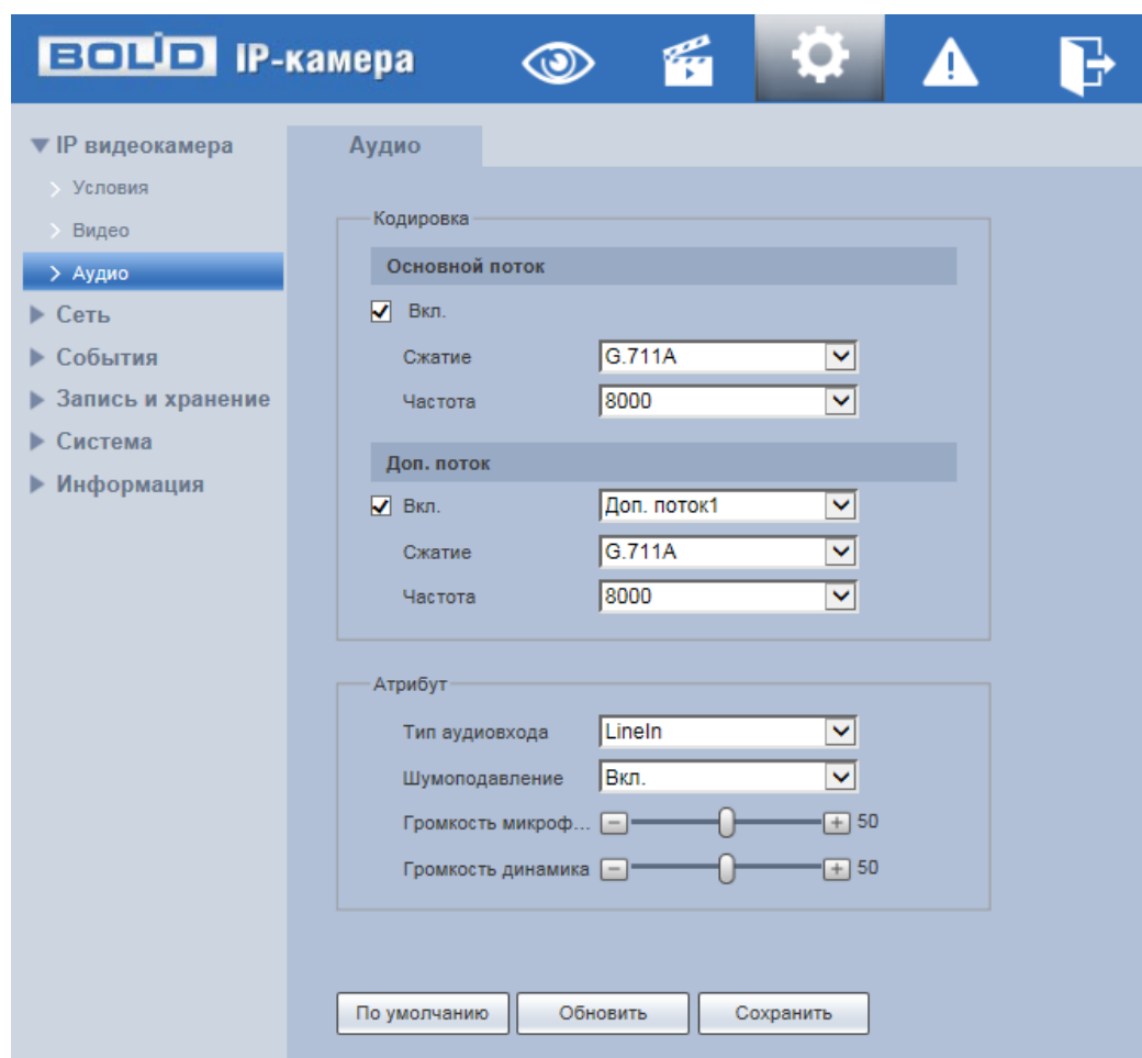
Рисунок 7.49 – Подпункт меню «Аудио»
