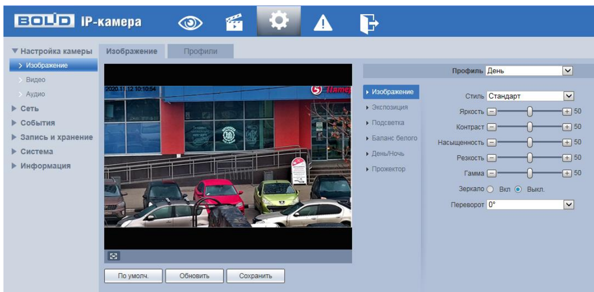
Рисунок 7.27 – Вкладка «Изображение»
