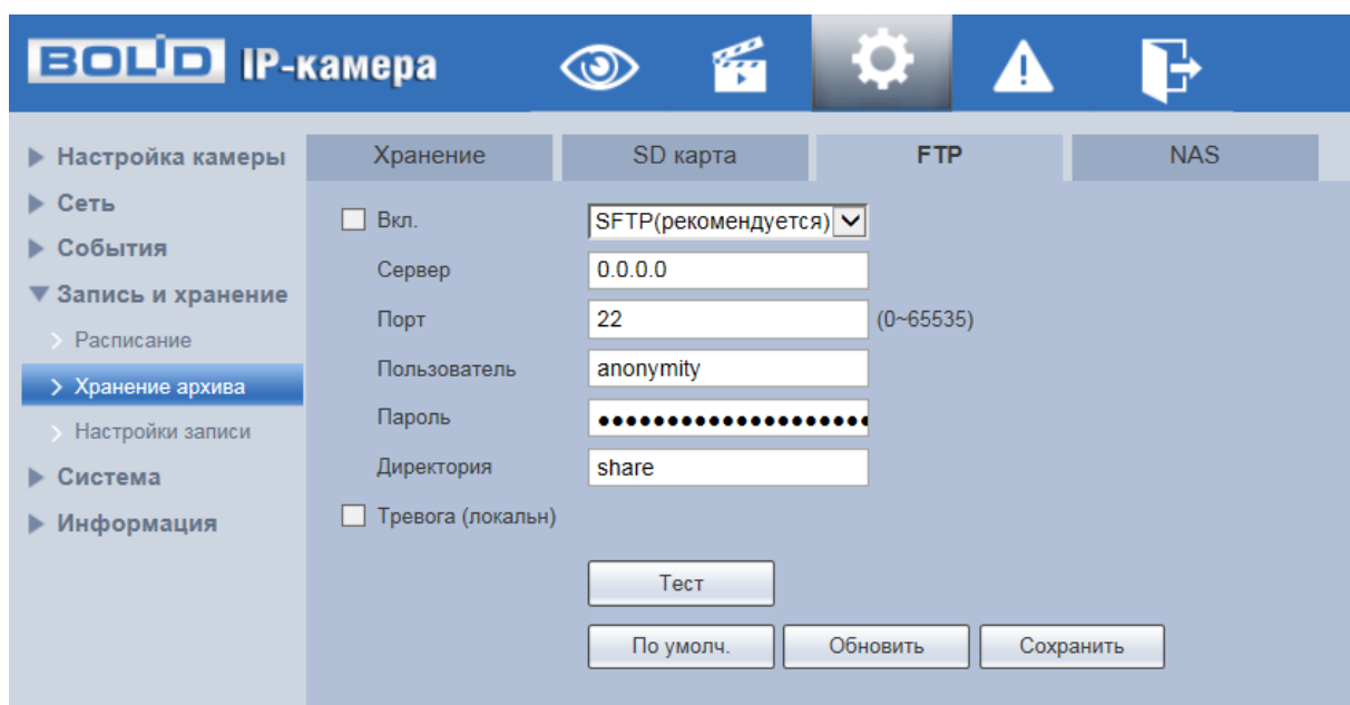
Рисунок 7.103 – Вкладка «FTP»
