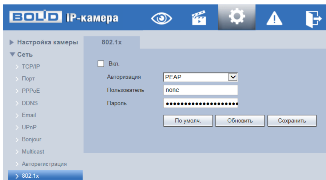
Рисунок 7.64 – Подпункт меню «802.1x»
