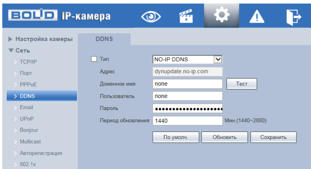
Рисунок 7.55 – Подпункт меню «DDNS»
