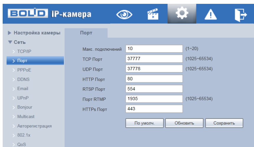
Рисунок 7.53 – Подпункт меню «Порт»
