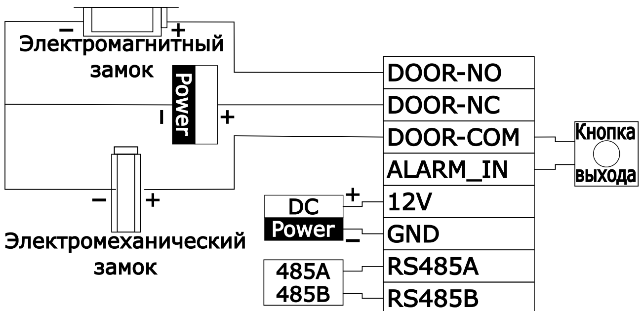
Рисунок 3.4 – Схема подключения. Замок 1
