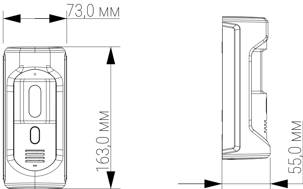
Рисунок 4.1 – Габаритные размеры
