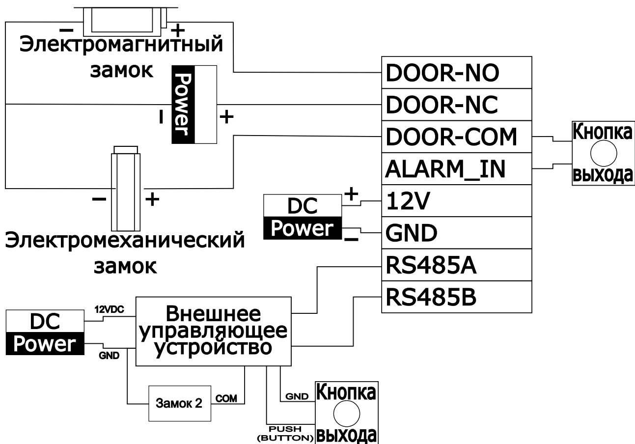
Рисунок 3.5 – Схема подключения. Замок 2
