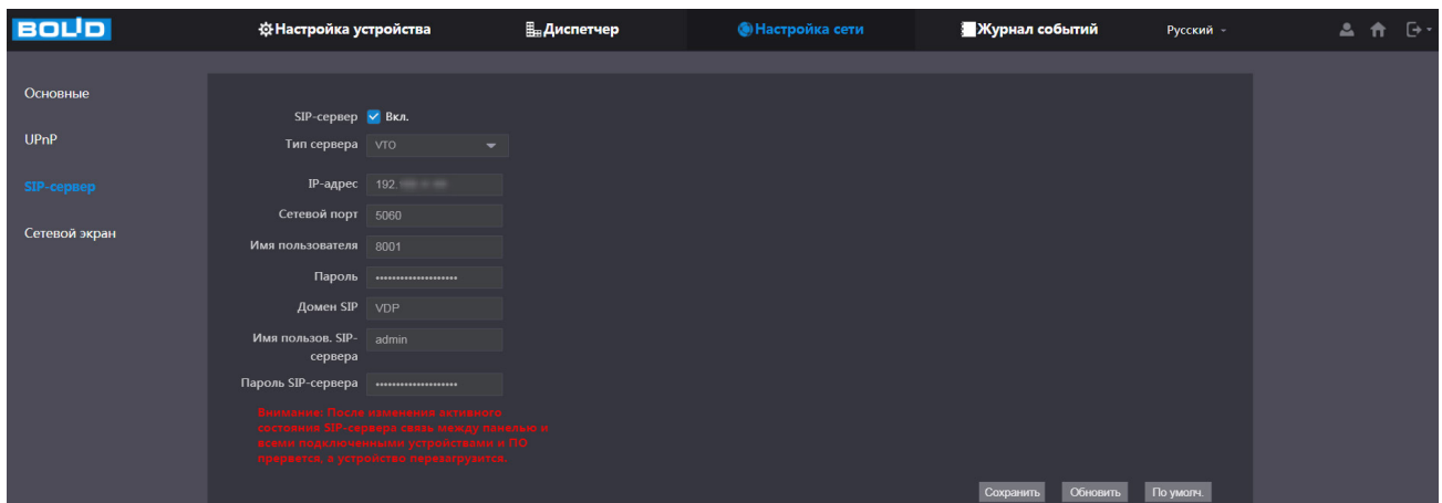
Рисунок 10.12 – Настройка SIP-сервера
