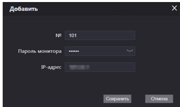
Рисунок 9.7 – Интерфейс добавления
