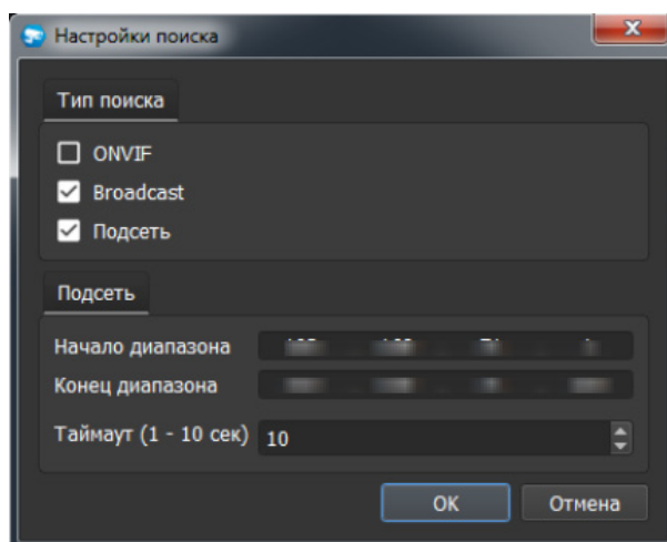
Рисунок 6.4 – Настройка поиска
