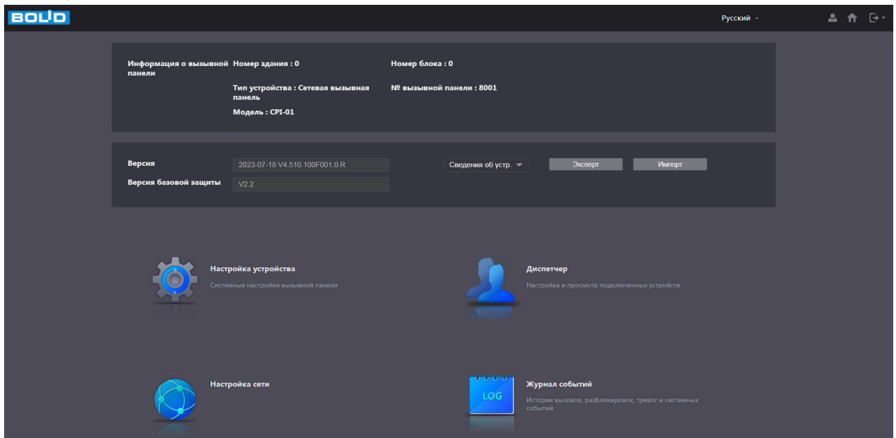
Рисунок 7.1 – Главное меню
