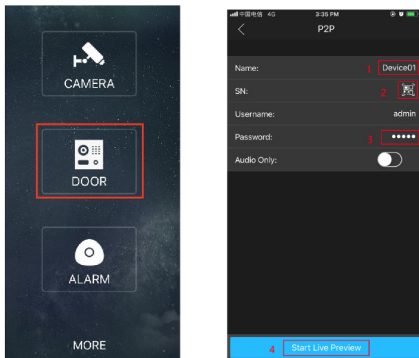
Рисунок 10.6 – Меню устройства
