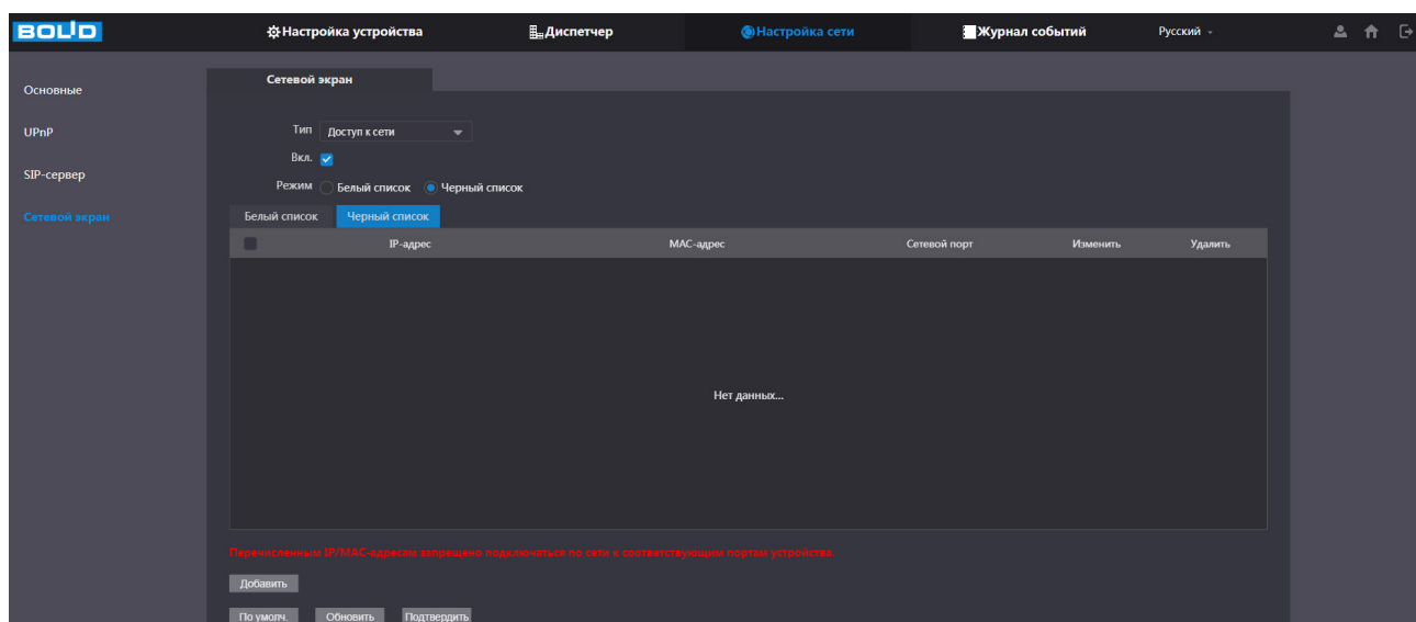
Рисунок 10.14 – Интерфейс настройки
