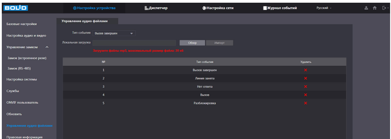
Рисунок 8.12 – Управление файлами
